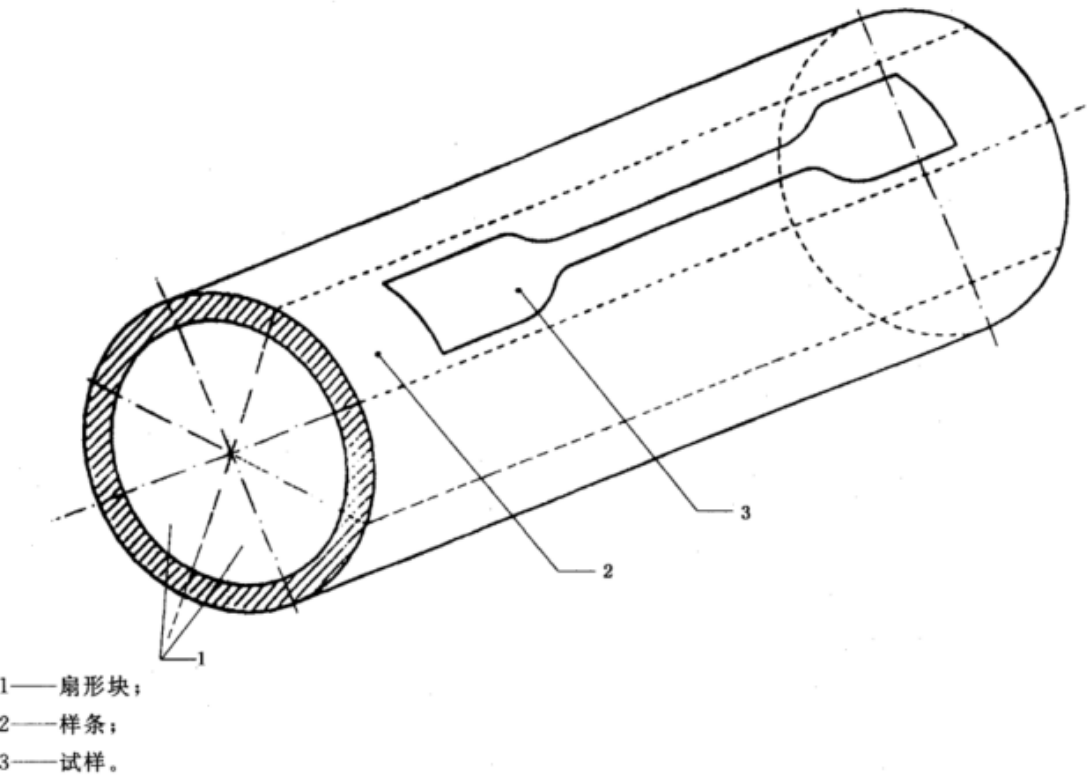
图 1 试样制备
